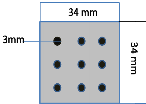
Fig. 3 Benchmark dimensions
