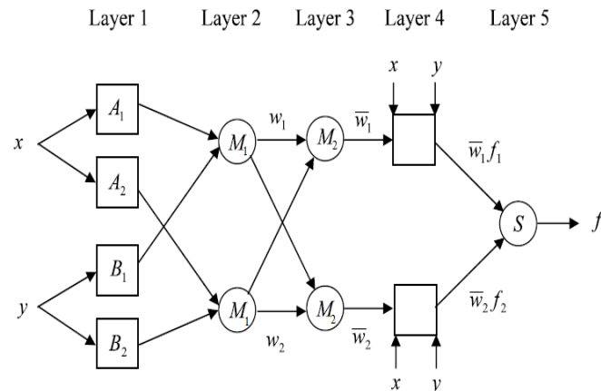
Fig. 3 ANFIS network
